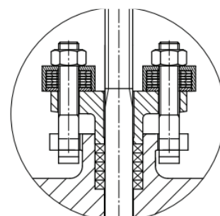
Federbelastete Stopfbuschpackung Spring loaded stuffing box
