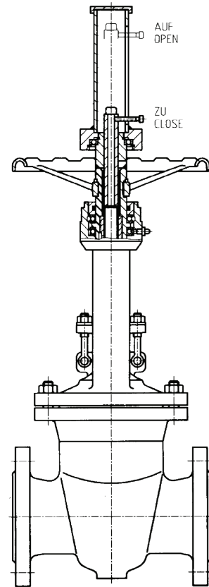
Ausführung mit Hubanzeige Design with stroke indicator
