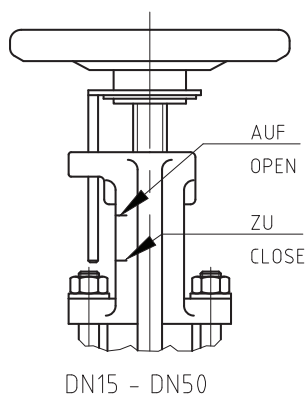
Ausführung mit Hubanzeige Design with stroke indicator
