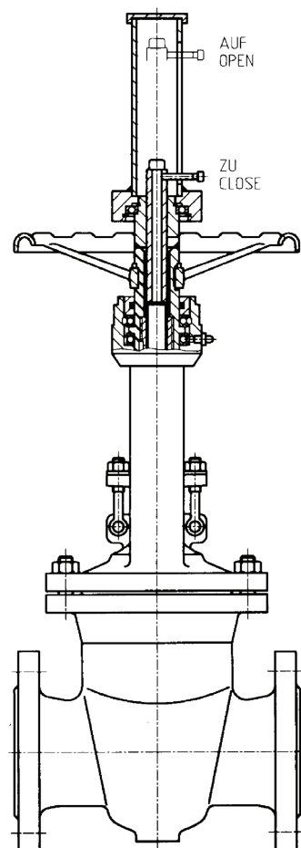
Ausführung mit Hubanzeige Design with stroke indicator
