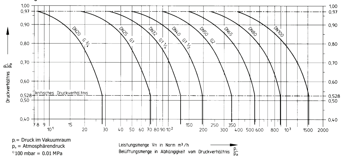
Leistungsdigramm Performance diagram
