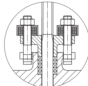
Federbelastete Stopfbuschpackung Spring loaded stuffing box
